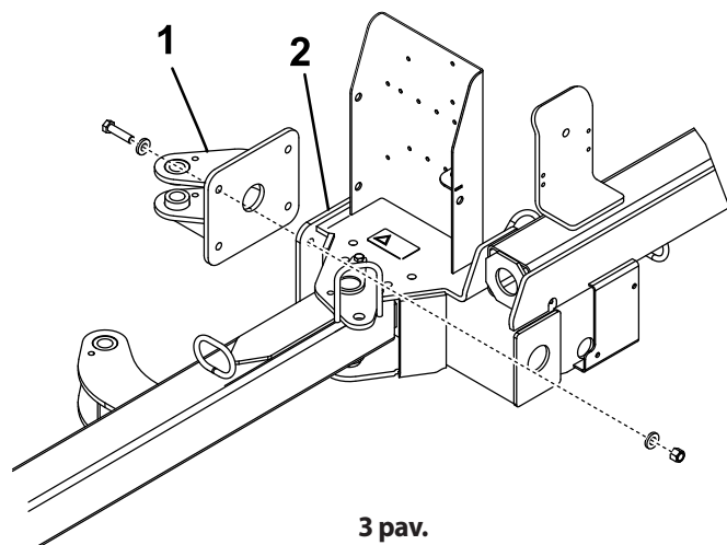
1. Galinės pavaros ąsa
